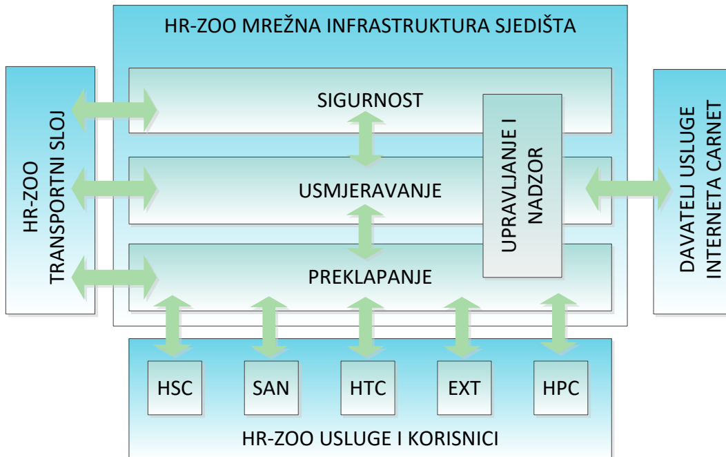
Slika 3: Pregled DC LAN-a
